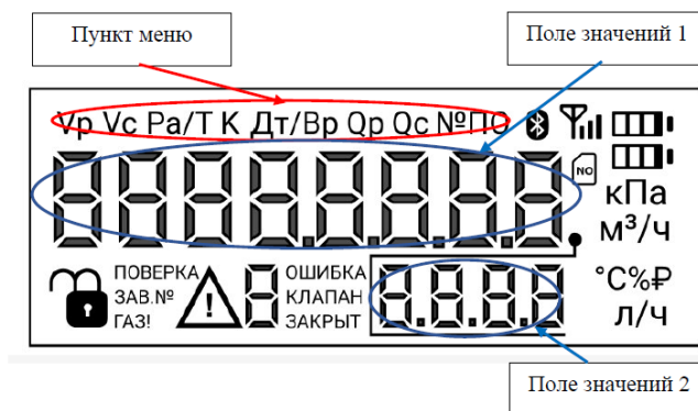
Рисунок 3 - Структура локального дисплея
