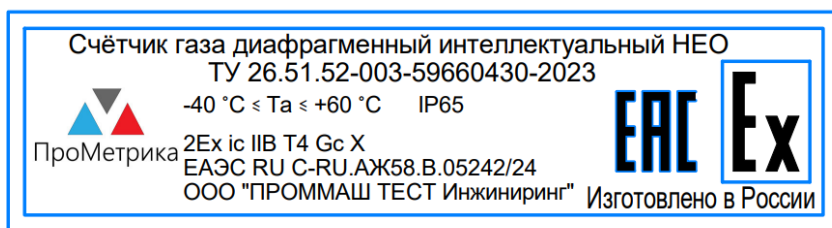
Рисунок 6 – Шильдик на боковой поверхности корпуса
