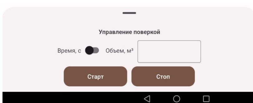
Рисунок 20 – Окно «Управление поверкой» мобильного приложения ПО «НЕО-Газ»
